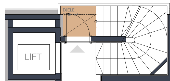
1.OBERGESCHOSS
