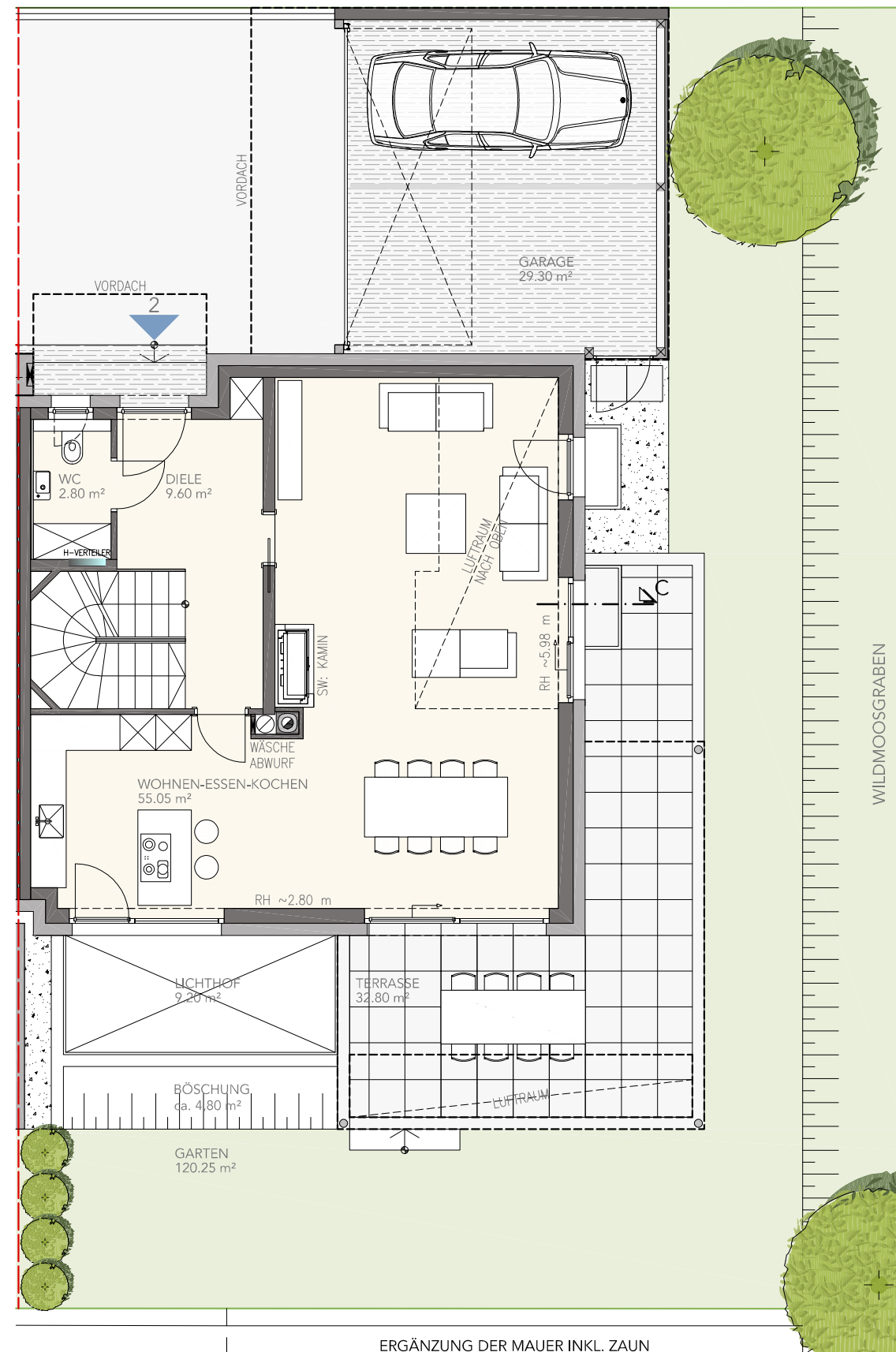
ERDGESCHOSS
