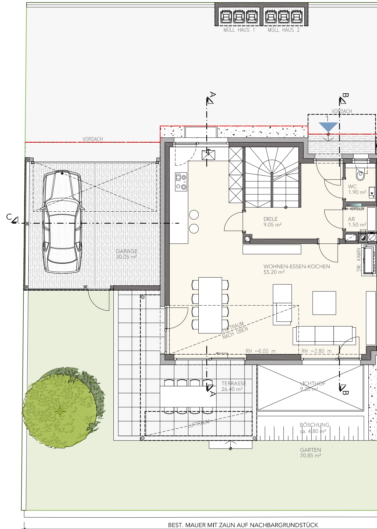
ERDGESCHOSS
