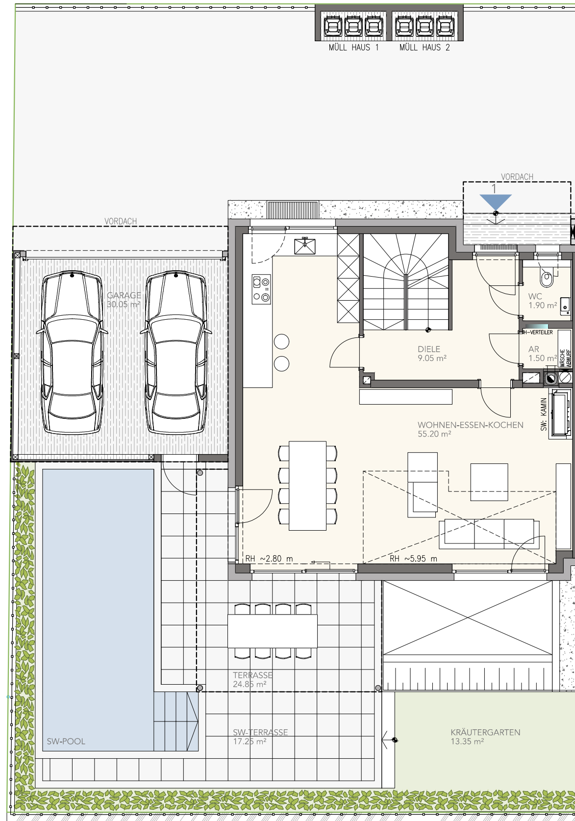
ERDGESCHOSS
